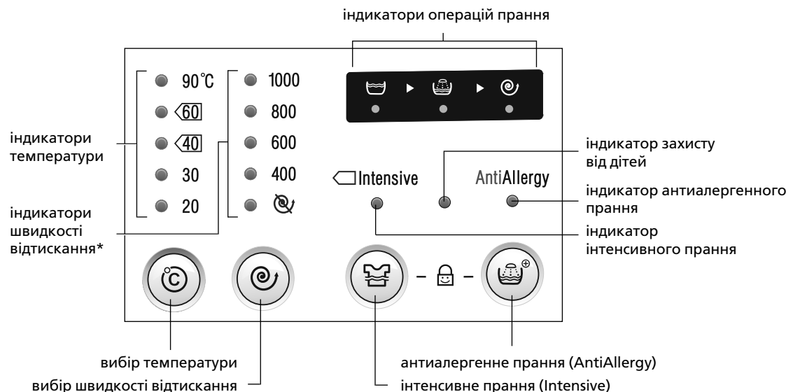
Рисунок 1 – Панель керування
