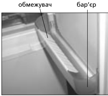
Рисунок 4 - Обмежувач
